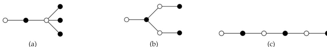
FIGUUR 4: Die drie 0-stabiele bome van orde 6.
