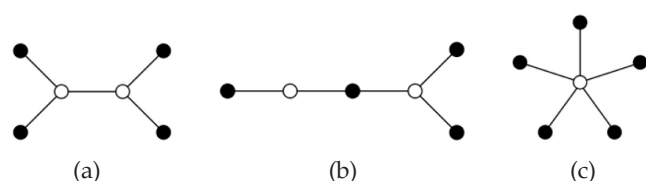
FIGUUR 1: Drie bome van orde 6 waarvan die onafhanklikheidsgetalle nie deur enkele lynverwyderings beïnvloed word nie. Maksimale onafhanklike versamelings word deur soliede punte aangedui.
