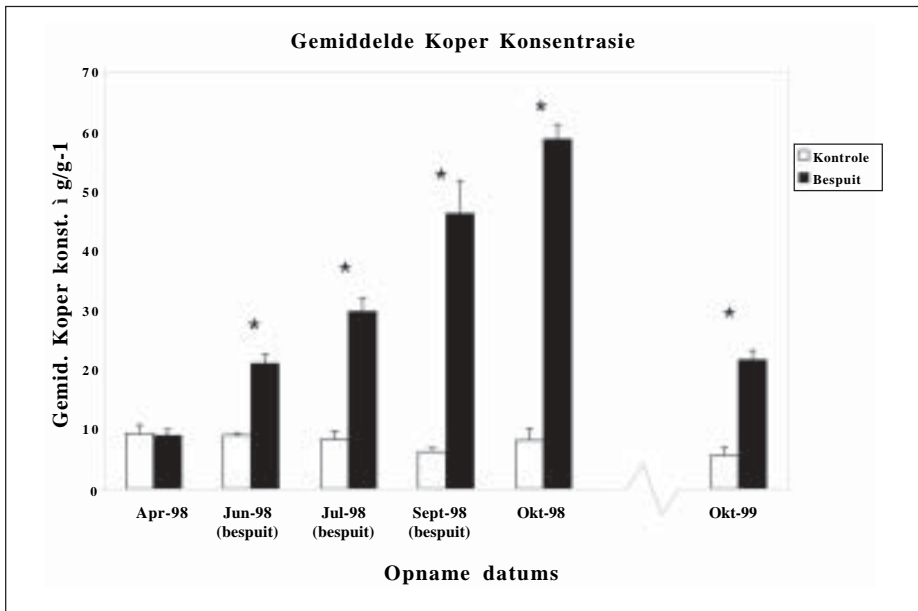
Figuur 3: Veranderinge oor verskeie maande in die koperkonsentrasies in die grond van die bespuite en kontrolepersele waar die invloed van die swamdoder, koperokschloried op die inheemse erdwurm Microchaetus sp. bestudeer is. * dui betekenisvolle verskille aan ( p < 0.05 ). (Uit: Maboeta et al 24 ).
